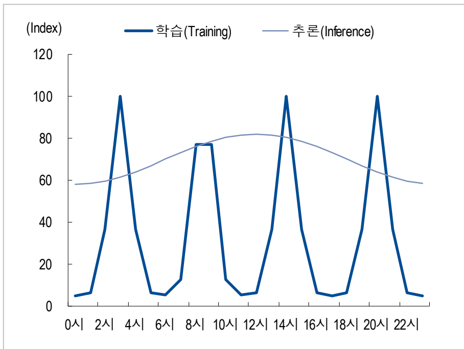
학습 vs 추론 전력 부하 프로파일
